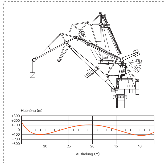
↑ Lenkersystem – horizontaler Lastweg
